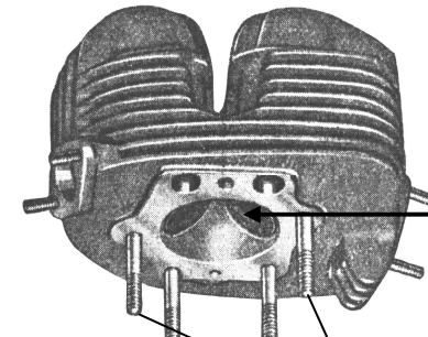
1281-1 Szpilki głowicy M10
