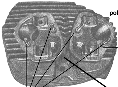
1281-2 Szpilki pokryw zaworowych
